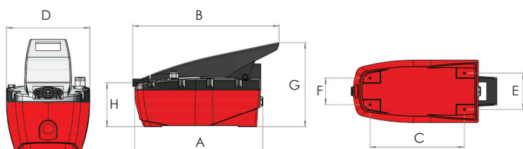
AHP1120 (serbatoio in plastica)
