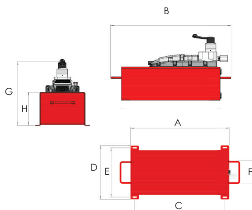
AHP1122, AHP1142 (serbatoio in acciaio)
