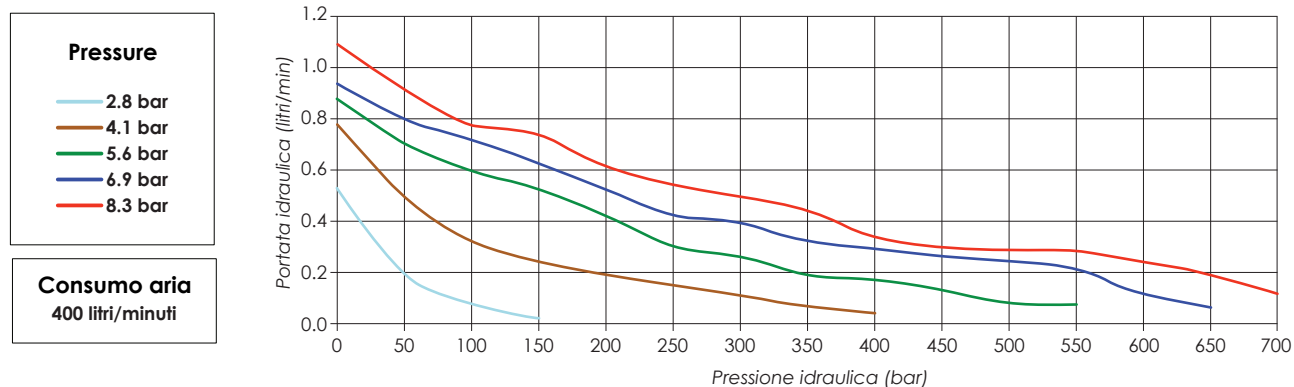
AHP1120 (serbatoio in plastica)
