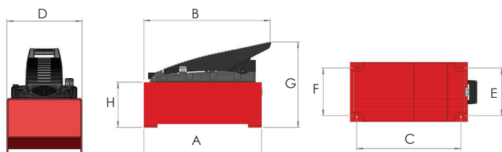
AHP1121, AHP1141 (serbatoio in acciaio)
