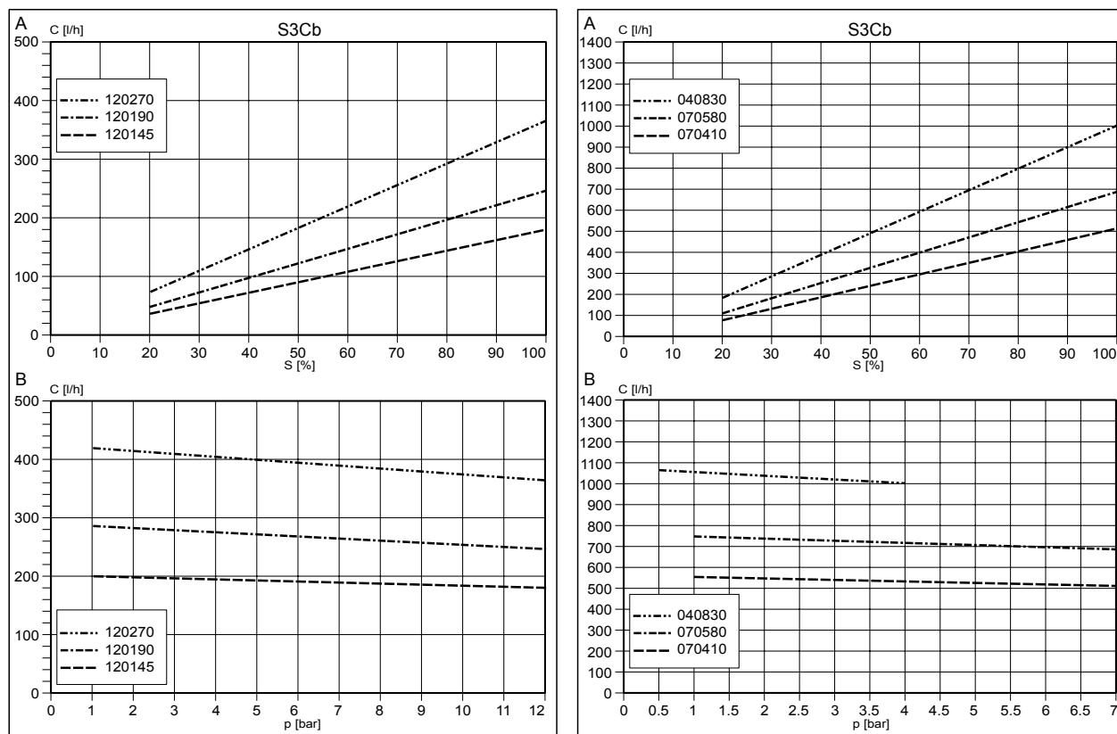
Fig. 1: A) Rendimento di dosaggio C con contro pressione minima in funzione della lunghezza corsa s . B) Rendimento di dosaggio C in funzione della contro pressione p .
